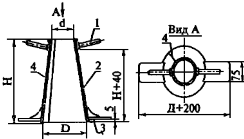
Рисунок 1 - Конус для определения подвижности
